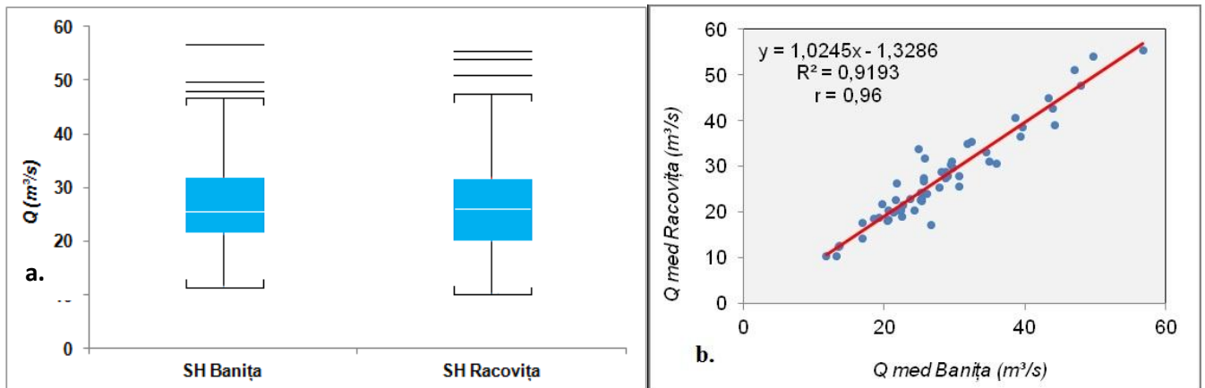
Figure 4. Diagramme box-plot (a) et corrélation statistique (b) des débits moyens annuels du Buzău enregistrés à Banița et à Racovița (1956-2011)
