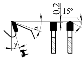
Рис. 1. Плоско-треугольный профиль зубьев с вогнутой передней гранью
