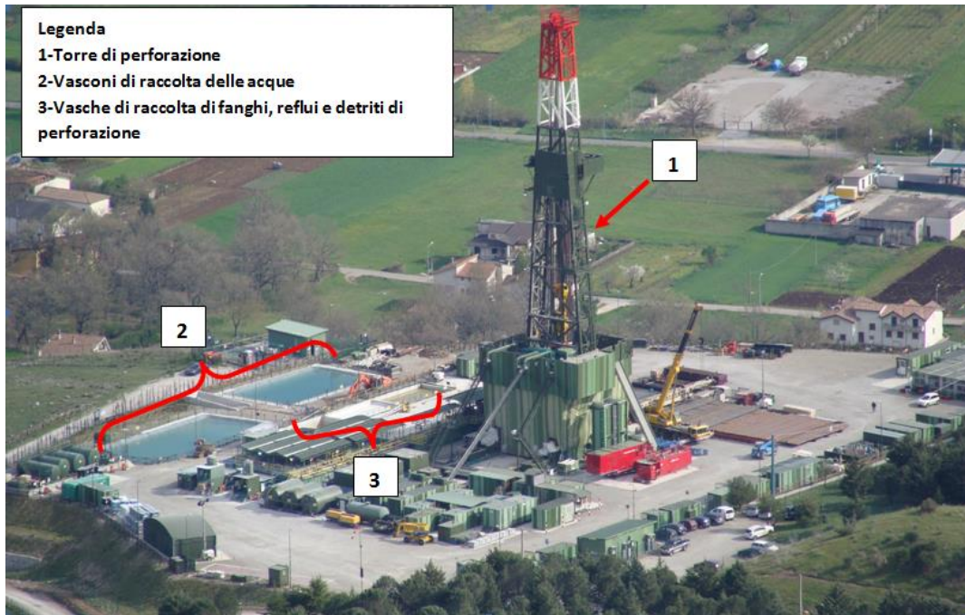
Fig. 2.11 Veduta del cantiere di perforazione del pozzo Alli 2, Marsicovetere (PZ)
