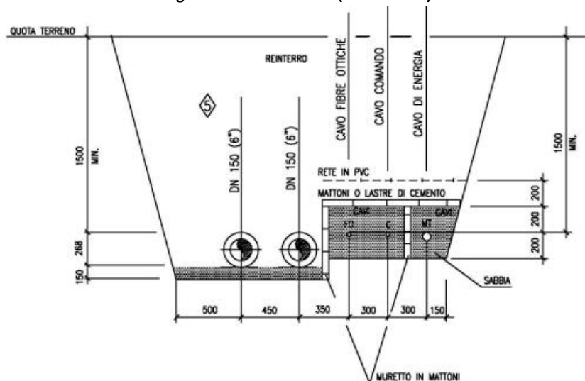
Fig. 1.1 Sezione di scavo (non in scala)
