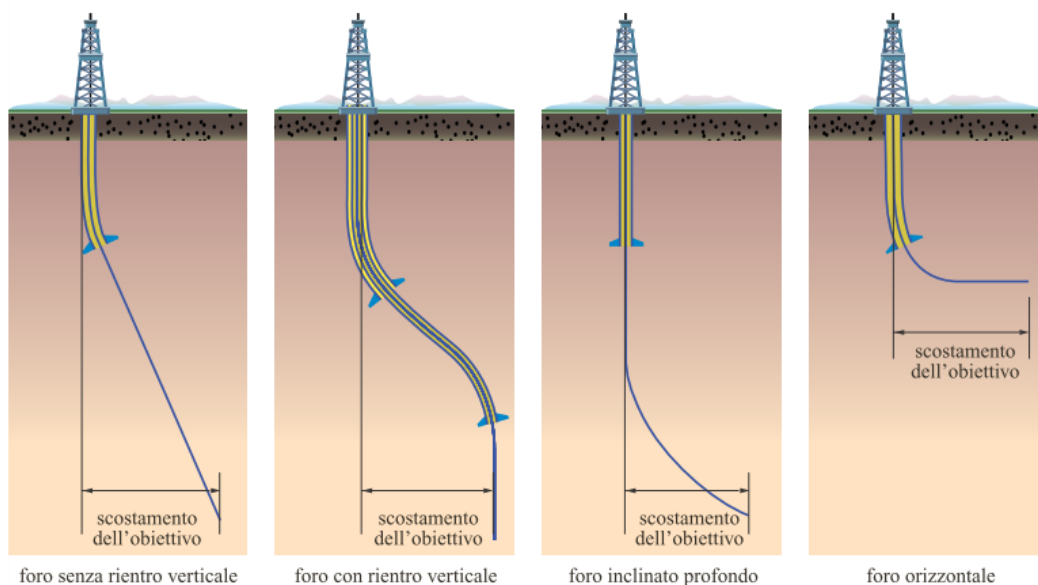
Fig. 1.6 Configurazioni principali che può assumere un pozzo direzionato od orizzontale
