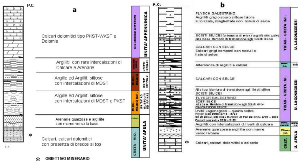
Fig. 2.1 Esempi di stratigrafie (a) e (b) di pozzi perforati nella concessione "Val d'Agri"
