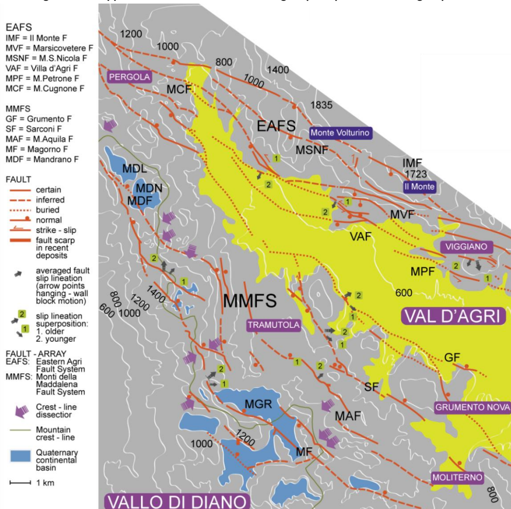
Figura 3.6 Mappa morfostrutturale della Val d'Agri: i principali sistemi di faglia quaternari
