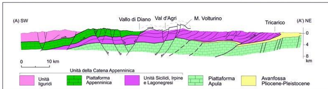
Figura 3.3 Sezione geologica regionale dell'Appennino Meridionale
