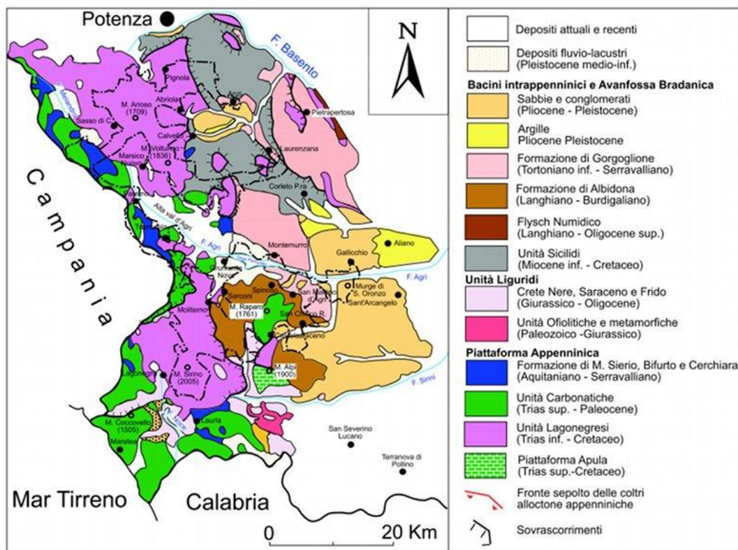
Fig. 3.4 Carta geologica schematica del territorio a Sud di Potenza
