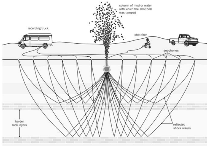
Fig. 1.2 Prospezione sismica con utilizzo di esplosivo
