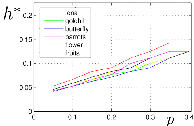
Fig. 10: Dependence of the optimal parameter h^* on p .
