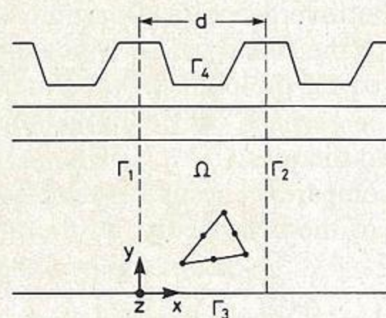
Fig. 1. Periodic waveguide.
