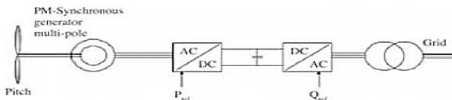
Figura 19. Esquema d'un aerogenerador.
