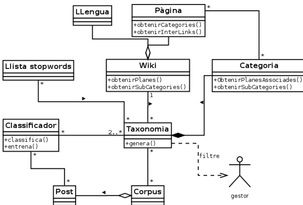
Figura 4.1: Diagrama de classes
