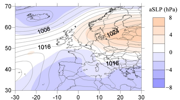
Figura 2: Composición del patrón sinóptico SLP correlacionado con el grupo IV
