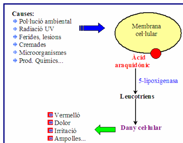
Figura 5.1. Procés d'inflamació.
