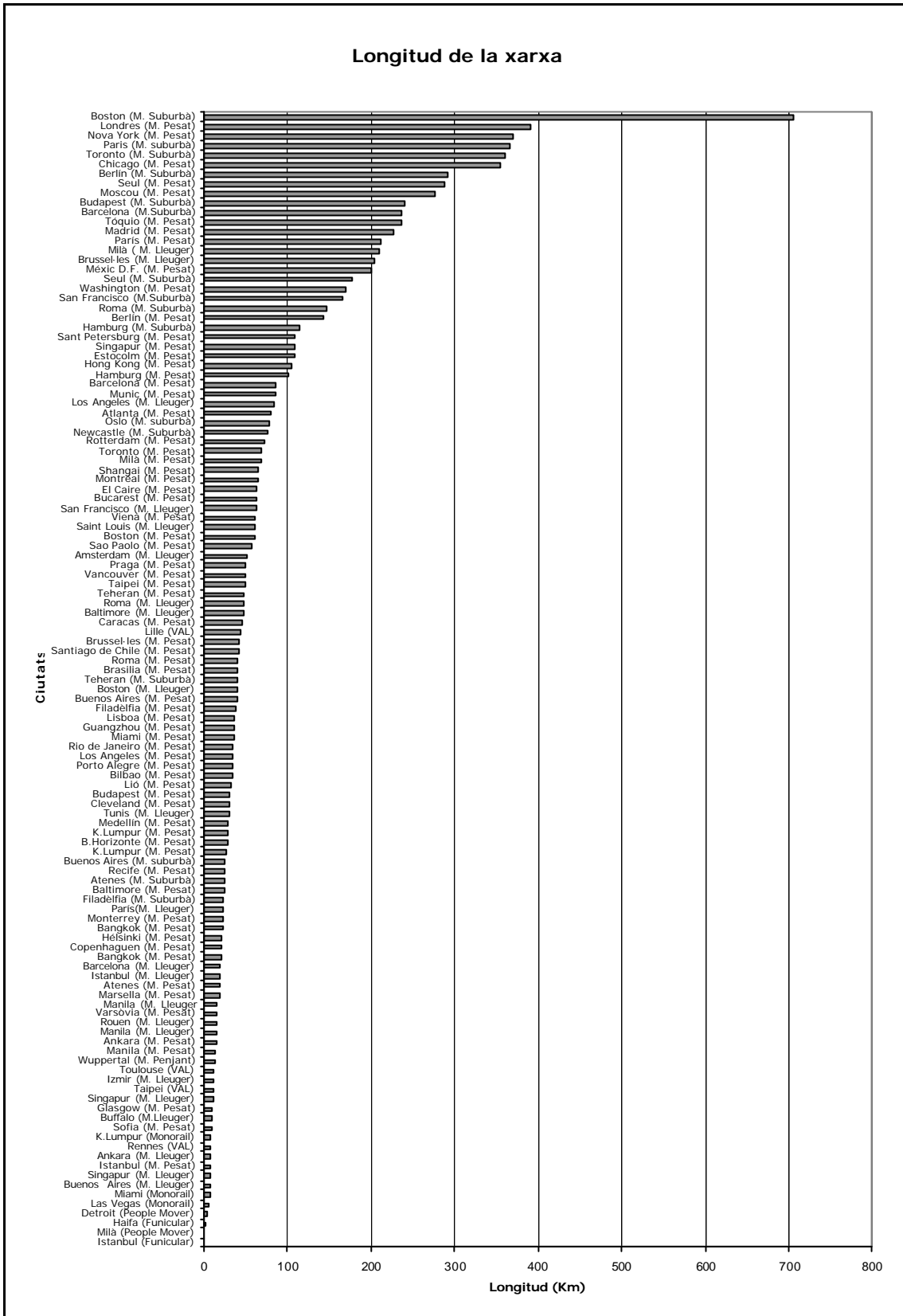
Figura C.8: Gràfica comparativa de la longitud de la xarxa de diferents sistemes ferroviaris metropolitans. Font pròpia
