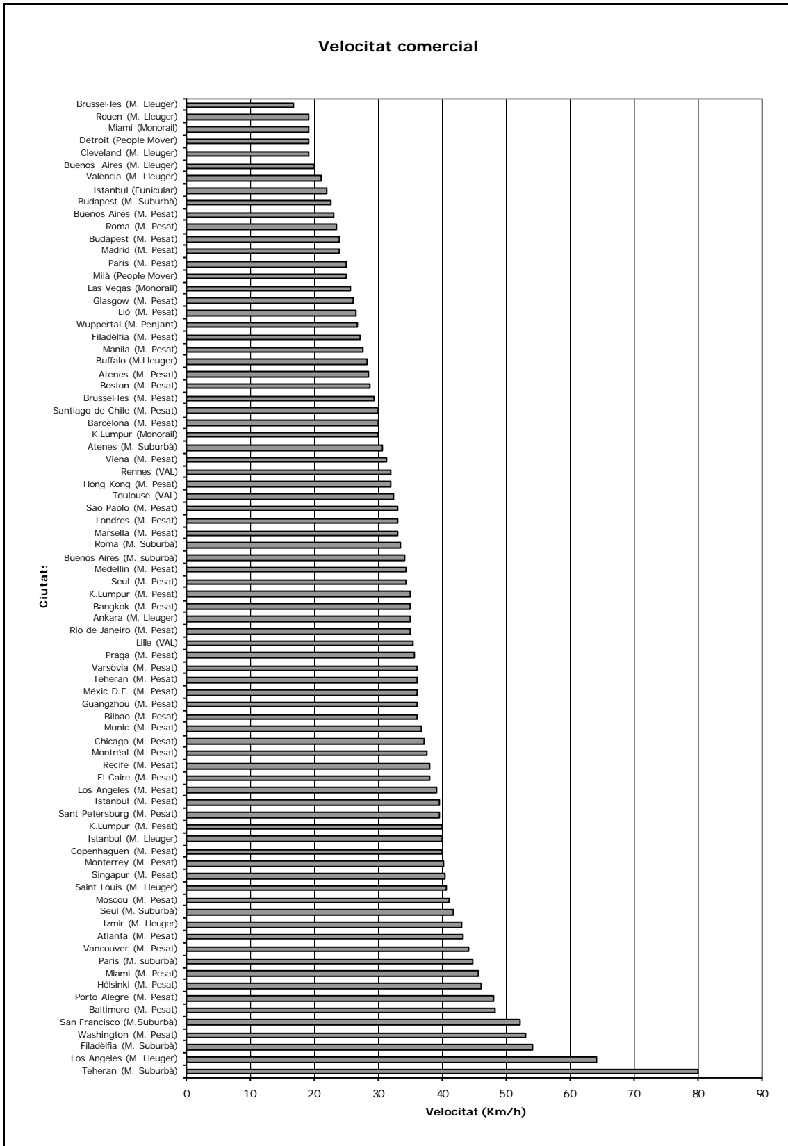
Figura C.5: Gràfica comparativa de la velocitat comercial de diferents serveis ferroviaris metropolitans. Font pròpia
