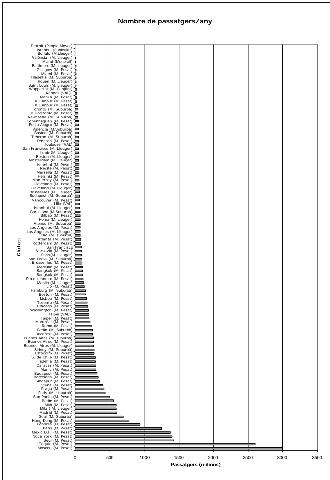
Figura C.10: Gràfica comparativa del nombre de passatgers/any de diferents sistemes ferroviaris metropolitans.
