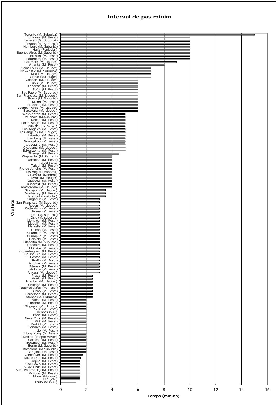
Figura C. 1: Gràfica comparativa d'interval de pas mínim de diferents serveis ferroviaris metropolitans. Font pròpia
