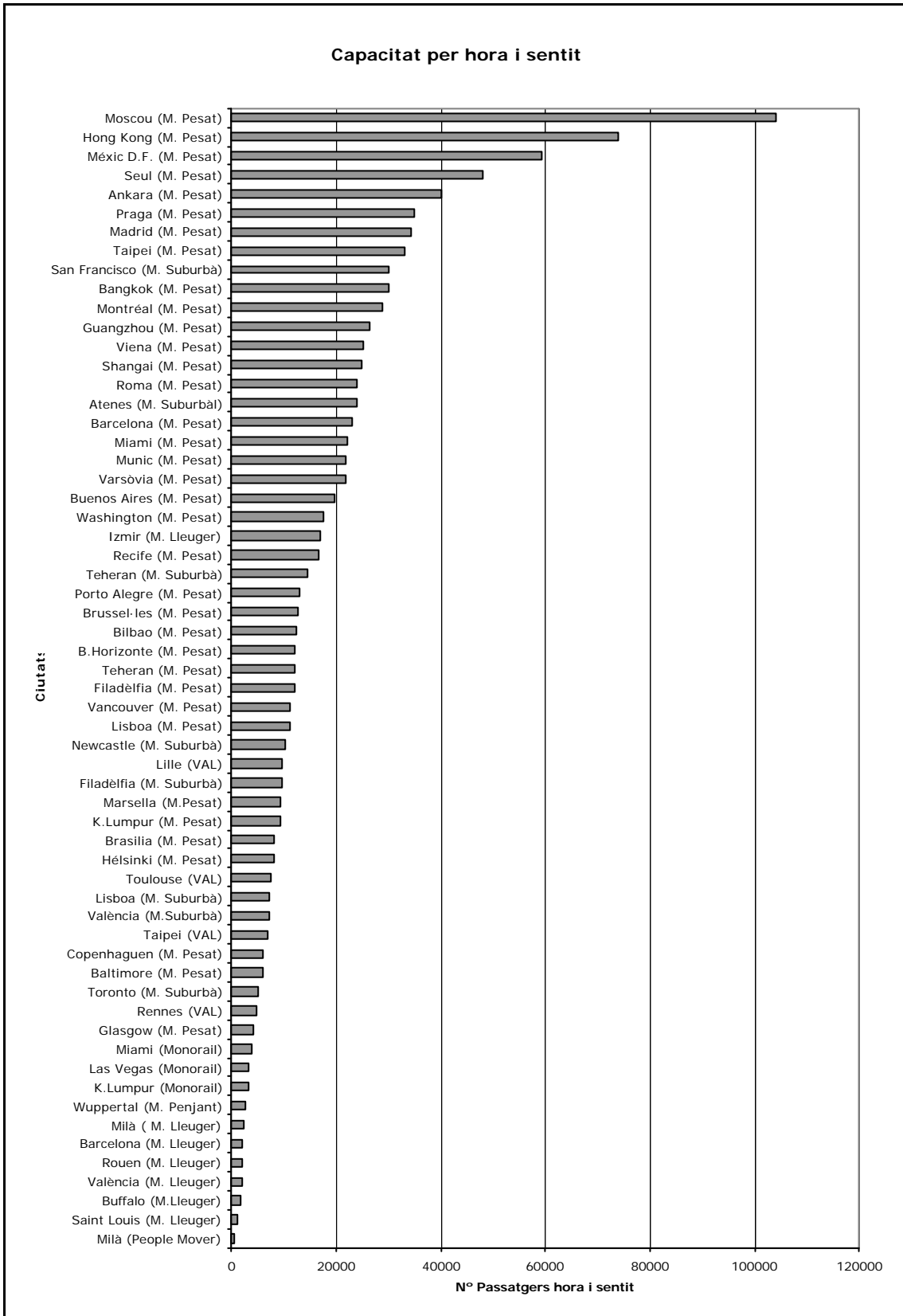
Figura C.4: Gràfic comparatiu de capacitat màxima de transport per hora i sentit de diferents serveis ferroviaris metropolitans. Font pròpia
