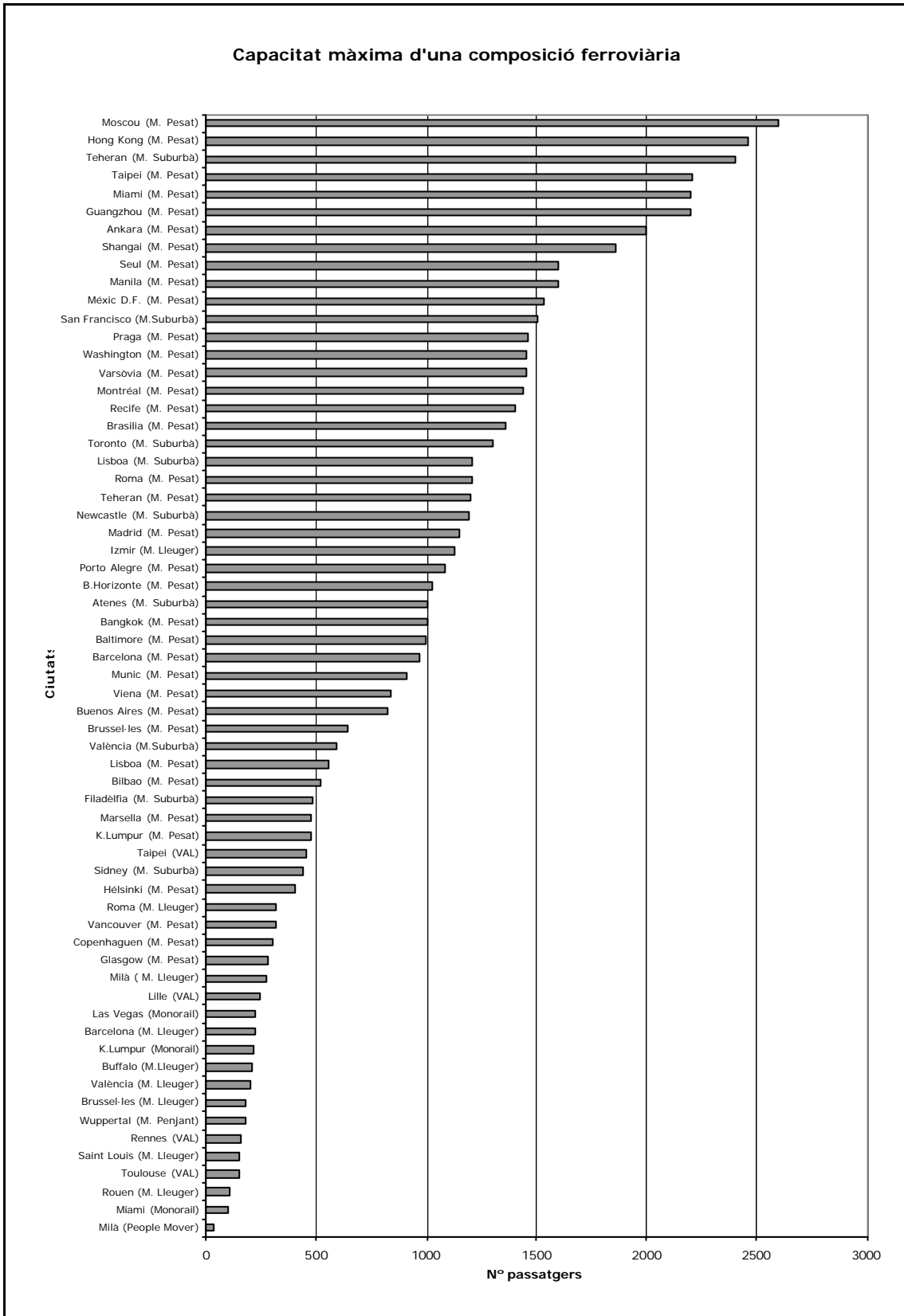
Figura C.2: Gràfica comparativa de capacitat màxima d'una composició ferroviària de diferents serveis ferroviaris metropolitans.
