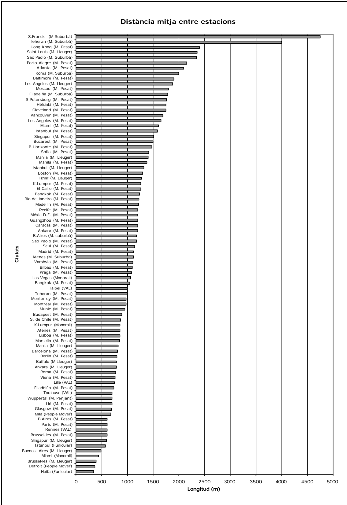
Figura C.6: Gràfica comparativa de distància mitja entre estacions de diferents serveis ferroviaris metropolitans. Font pròpia
