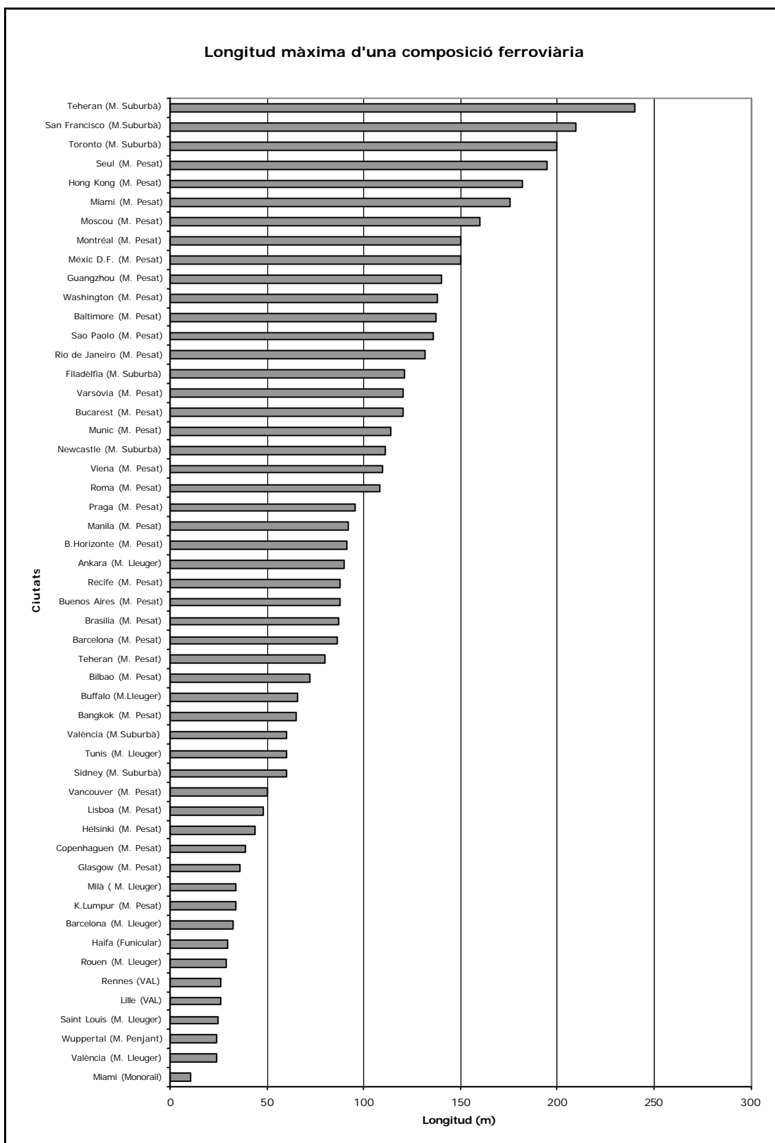
Figura C.3: Gràfica comparativa de longitud màxima d'una composició ferroviària de diferents serveis ferroviaris metropolitans.
