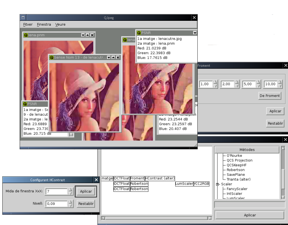
Figura 4.2: Mostra de les principals finestres del programa. La principal, amb versions de la imatge a restaurar. A sota, la cadena de descodificació. A dalt a la dreta, de fons, la configuració de la baula de Froment. A l'esquerra, configuració de la baula HContrast.
