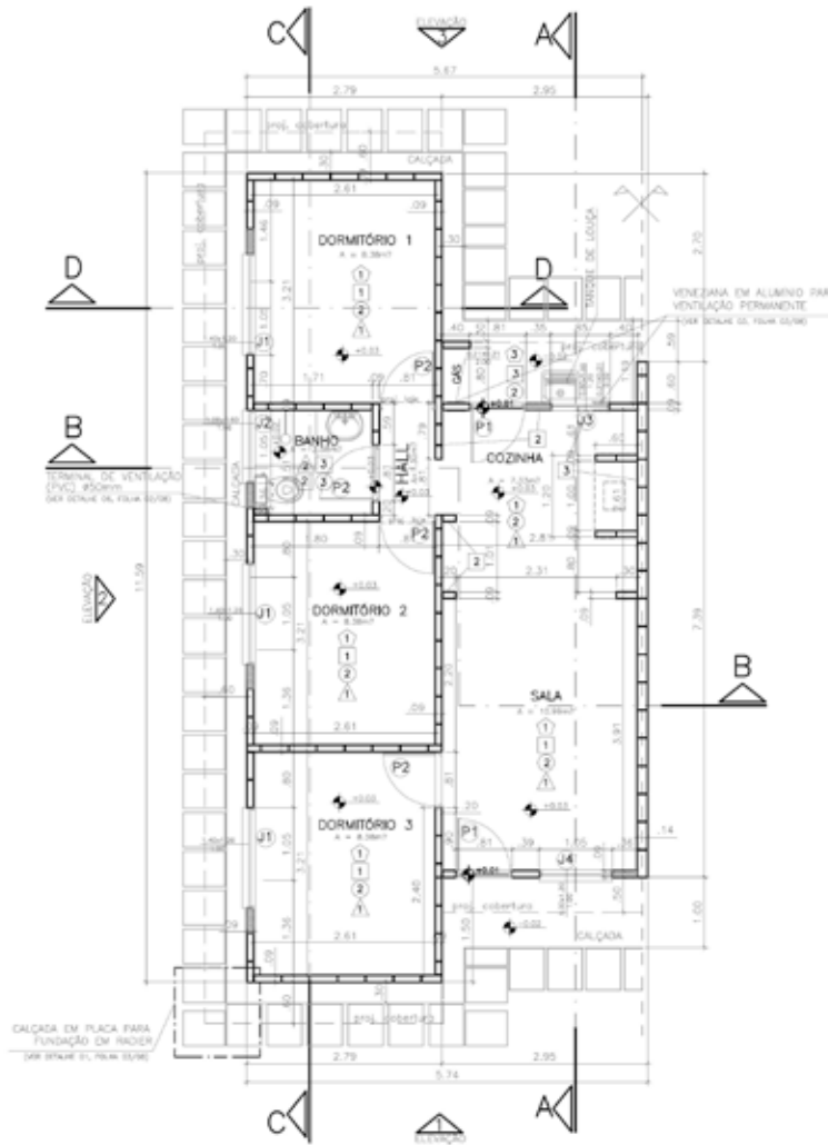
Fig. 3 - Planta da tipologia TG23A com opção de 3 dormitórios (CDHU)
