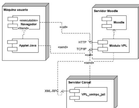
Figura 1. Arquitectura de los componentes software
