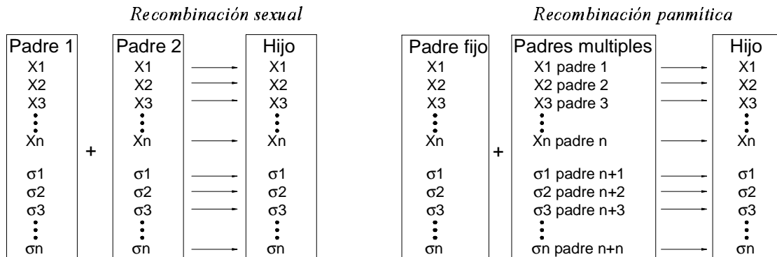
Figura 1. Esquemas básicos de recombinación en Estrategias Evolutivas
