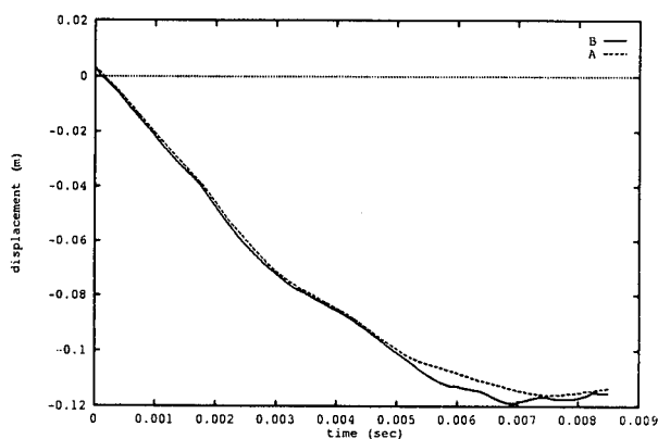
Figura 12. Posição dos nós A e B (m) durante impacto
