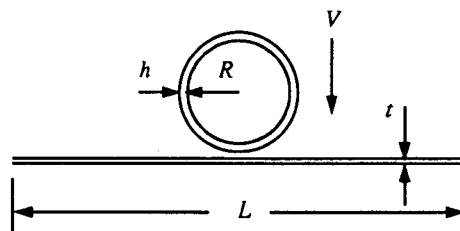
Figura 7. Geometria da placa e tubo: R = 0.097 \text{ m} ; h = 0.006 \text{ m} ; L = 1.2 \text{ m} ; t = 0.003 \text{ m}
