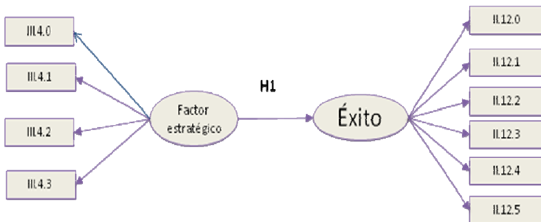
Figura 1: Relación causal entre el factor estratégico y el éxito del proyecto
