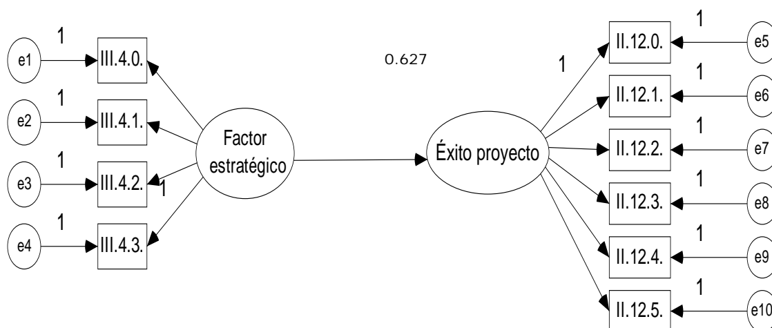
Figura 2: Modelo estructural de las relaciones causales entre el factor estratégico y el éxito de proyecto de GC
