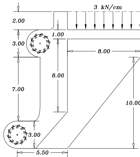
Figura 9. Forma inicial (cm) e condições de contorno: ( E = 21,0 \times 10^3 \text{ kN/cm}^2 ; \nu = 0,3 ; \rho = 7,81 \times 10^{-3} \text{ kg/cm}^3 )
