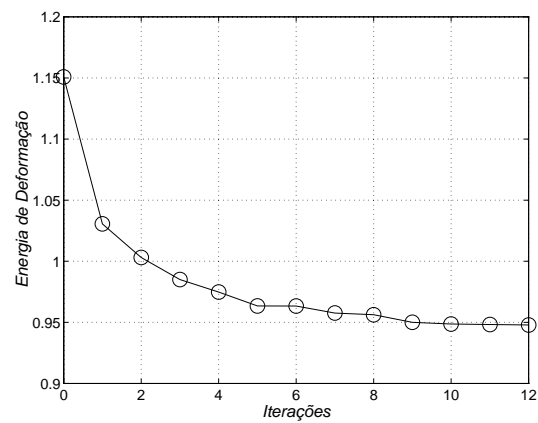
Figura 7. Energia de deformação durante as iterações
