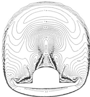
Figura 1.- Flujo de movimiento entornero lanzadera espacial [1]
