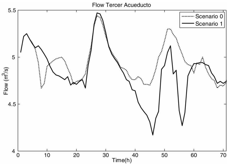
Figure 5 | Flow at Tercer Acueducto.
