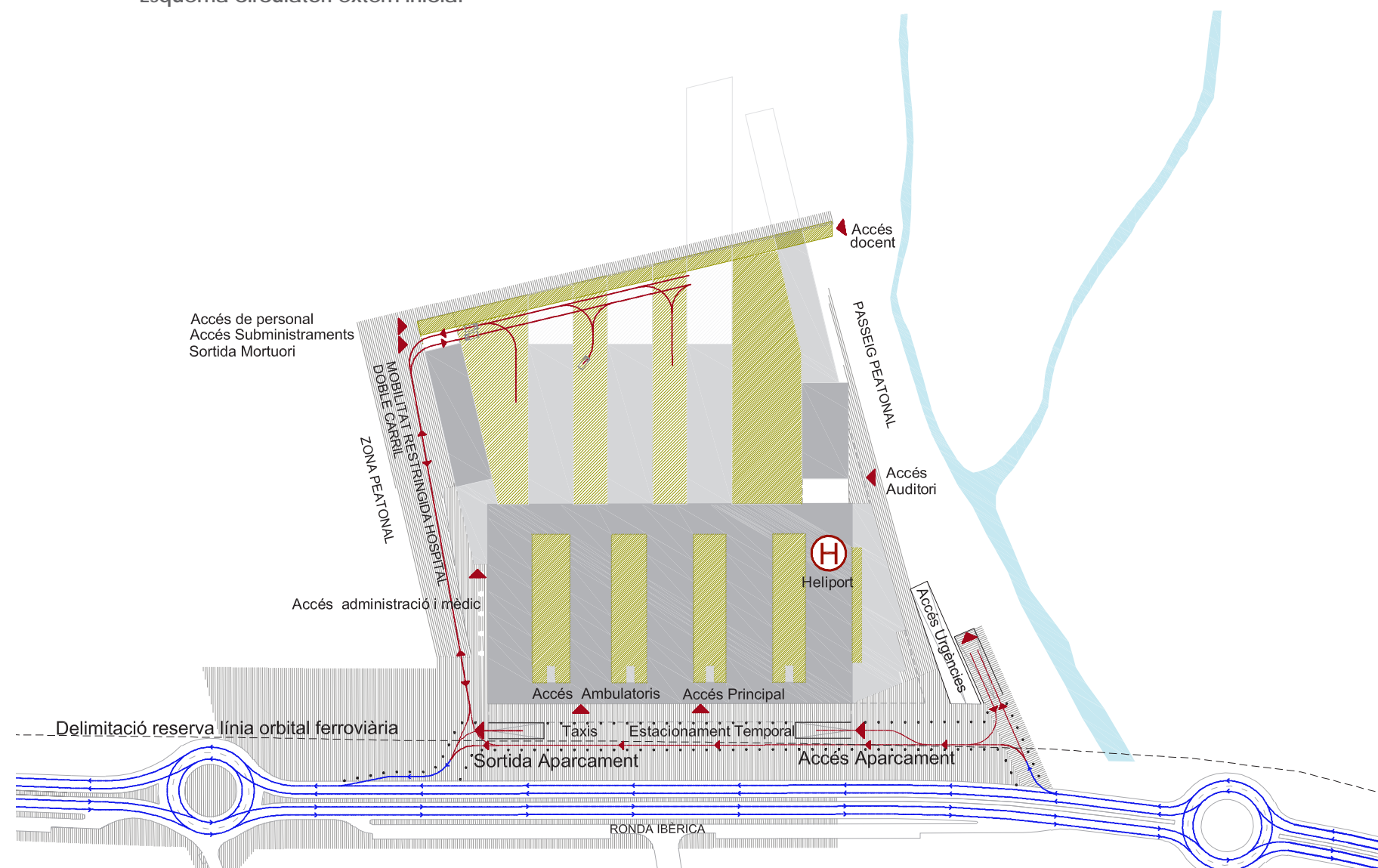
Esquema circulatori extern inicial
