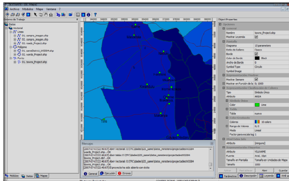
Figura 4: Interficie gráfica de SEXTANTE [6].
