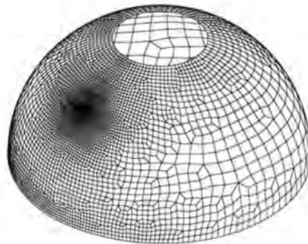
mesh 1: 2242 el 15.1%
