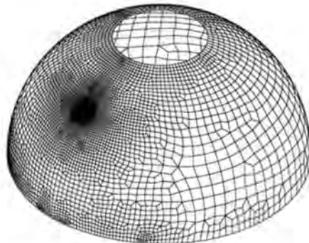
mesh 2: 2698 el 14.0%
