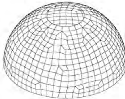
mesh 0: 320 el 59.2%
