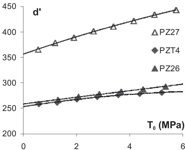
Fig. 7- Dependencia de d_{33} con la amplitud para distintos materiales.
