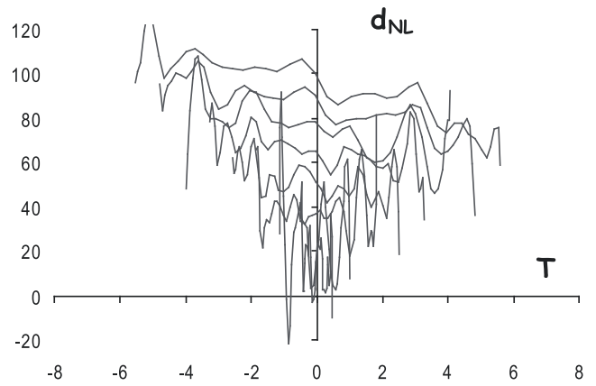
Fig. 2- El coeficiente piezoeléctrico d NL se obtiene a partir de la derivada de \bar{D} respecto a T. Se observa cómo depende no sólo de T, sino también de su amplitud T 0 .
