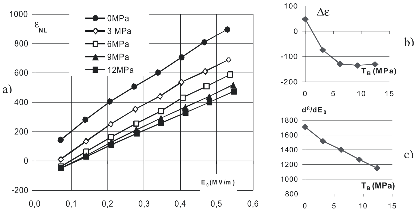
Fig. 6- a) Dependencia de la constante dieléctrica con la amplitud del campo E_0 y con T_B . b) Dependencia de la constante dieléctrica lineal con T_B . c) Dependencia de la pendiente de \epsilon(E_0) con T_B .
