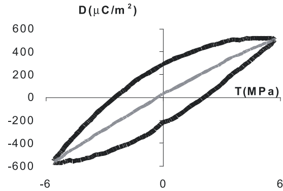
Fig. 1- a) Desplazamiento eléctrico D 3 en función del esfuerzo uniaxial instantáneo T 33 . Se muestra su valor medio \bar{D}
