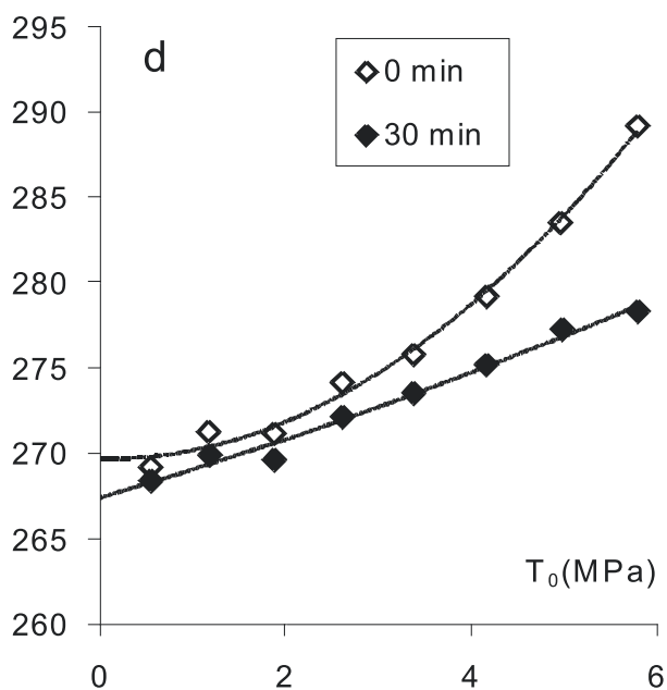
Fig. 4- Dependencia de d_{33} en función de la amplitud del esfuerzo según el tiempo transcurrido desde la aplicación del pre-esfuerzo.
