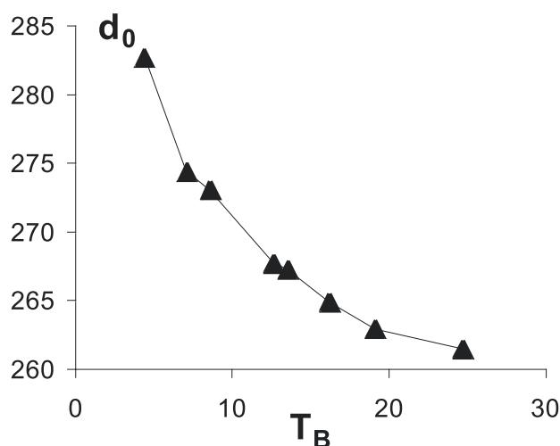
Fig. 5- Valor de d_0 ( d_{33} a amplitud T_0 nula) en función de T_B .
