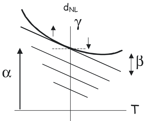
Fig. 3- Efecto de cada uno de los coeficiente sobre el aspecto de d_{NL}(T) : \alpha mide su desplazamiento, \gamma mide su inclinación, y \beta su curvatura.
