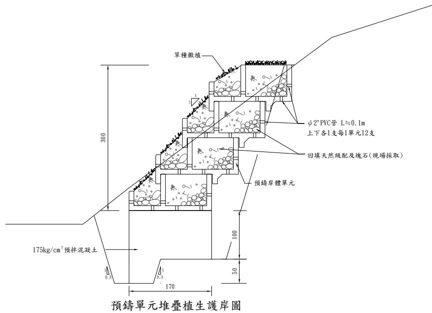
圖 8. 植生護岸標準圖
