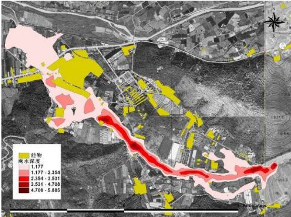
圖 5. 25 年重現期距模擬現況淹水深度示意圖
