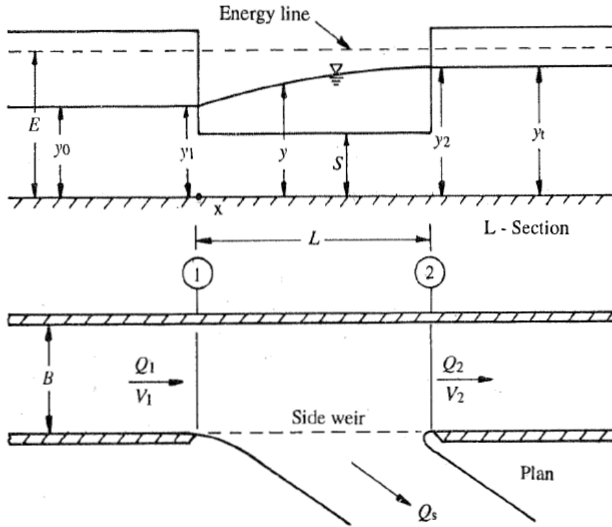
附圖 1. 側堰之示意圖(Subramanya, 2003)
