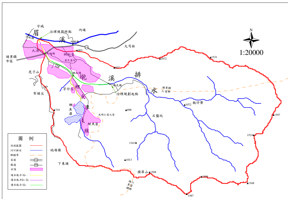
圖3. 墘溪排水現況通水能力示意圖
