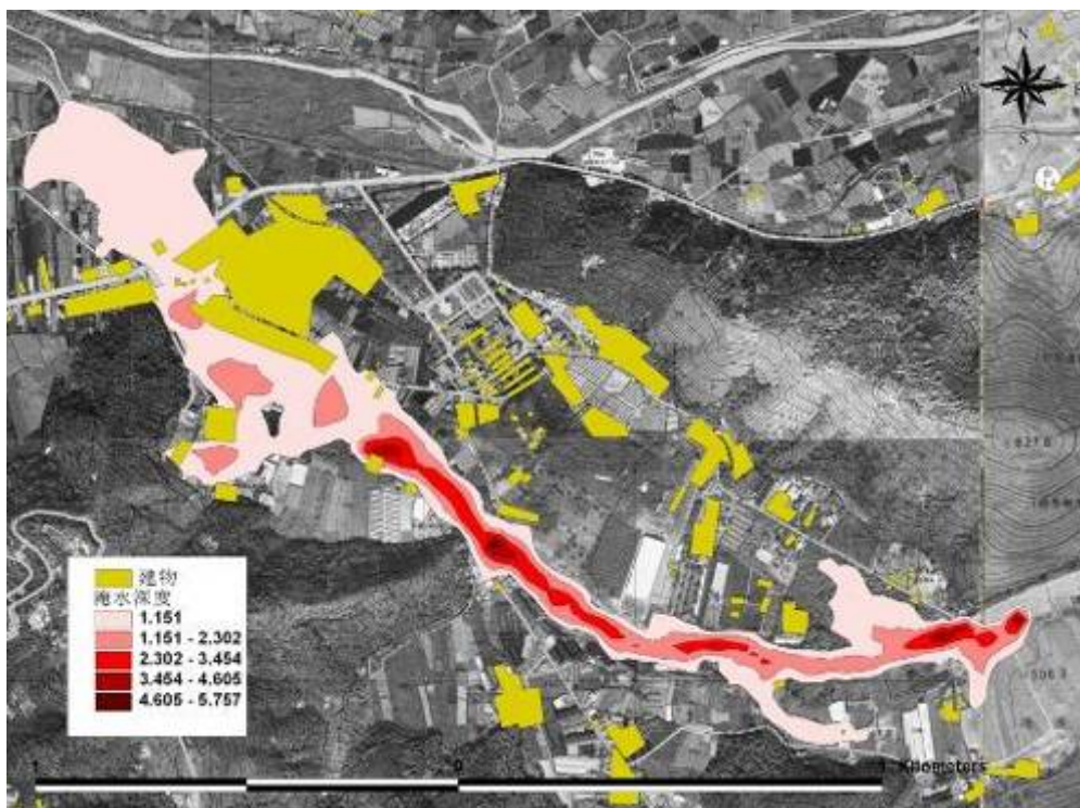
圖 4. 10 年重現期距模擬現況淹水深度示意圖
