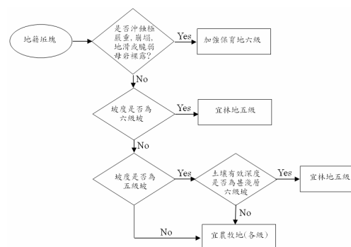
圖 3. 土地可利用限度分級流程圖 Figure.3 Slopeland land use classification flow chart
