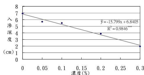
圖 5. 不同處理下之噴灑入滲深度
