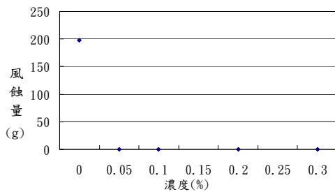
圖 7. 不同處理下風蝕損失量
