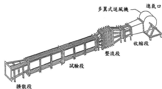
圖 4. 風洞簡圖
