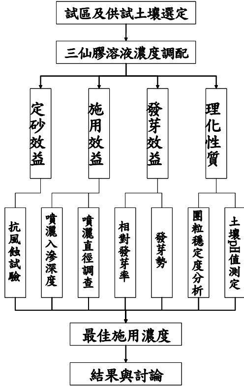
圖 1. 研究流程圖
