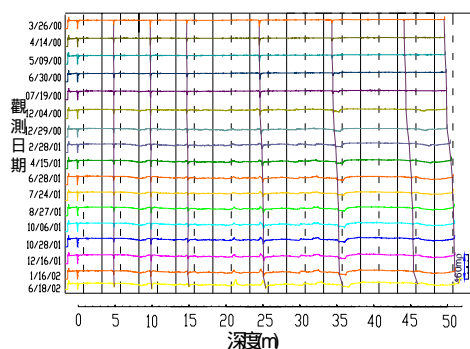
圖 4. C1 測站波形資料圖
