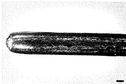
1 TENSION (cone)
