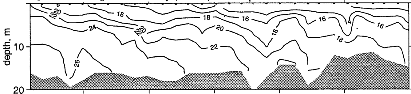
Figure 36a. Longitudinal Survey (8/17/95): Salinity Contour
