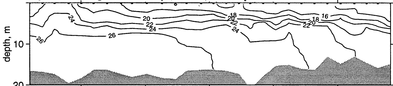
Figure 38a. Longitudinal Survey (10/18/95): Salinity Contour
