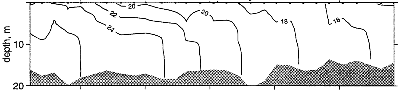
Figure 40a. Longitudinal Survey (10/22/95): Salinity Contour
