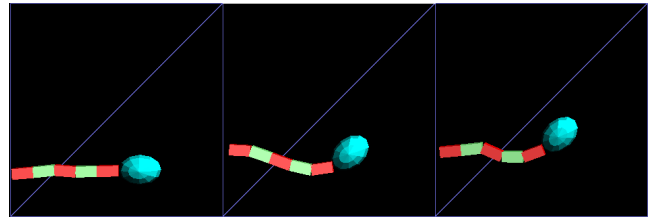
Fig. 8. Snake gait.
