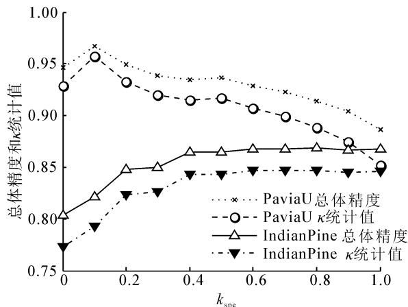
图 3 不同 k_{spe} 设定值下的分类结果
