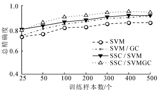
(c) Pavia University 数据集总体精度
