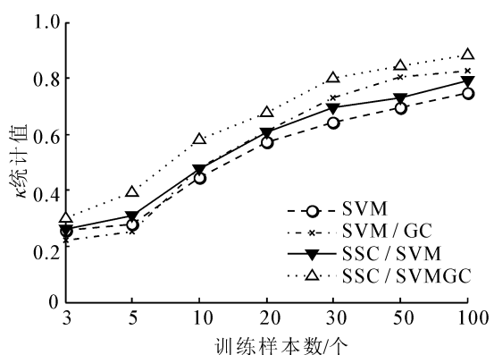
(b) Indian Pine 数据集 \kappa 统计值
