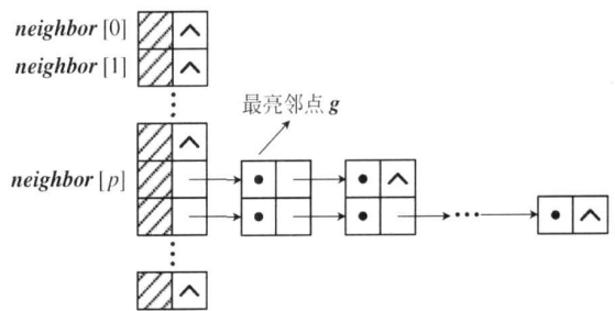
图 3 保存 N(S_m) 的链表数组
