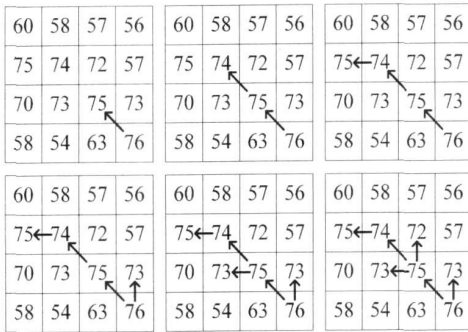
图 2 前 6 次迭代的结果
