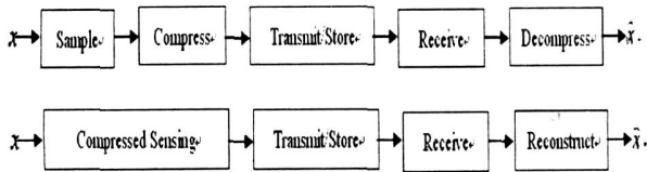
图 1 传统数据处理和 CS 数据处理的比较
