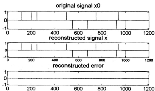
图 3 一维数据恢复
