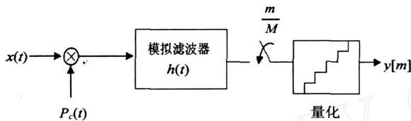
图 2 AIC 设计方案
