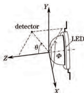
图2 \Phi 角和 \theta 角的定义
