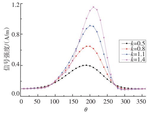
(b) 信号强度随着辐射阻尼相位 \theta 和不同增益倍数 K 之间的变化曲线
