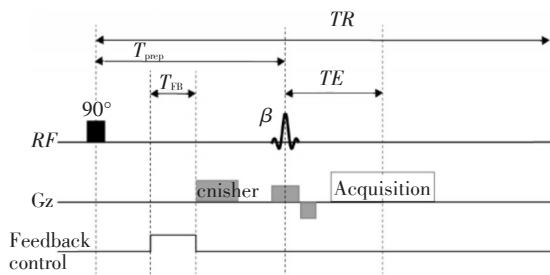
图3 正反馈增强模拟脉冲序列,在 90^\circ 硬脉冲作用后,正反馈系统持续 T_{FB} 时间,最后用一般成像序列观察成像信号
