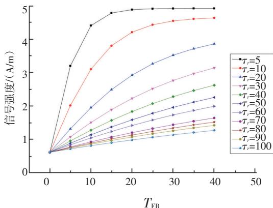
(a) 信号强度随着辐射阻尼作用时间 T_{FB} 在不同的辐射阻尼时间常数 \tau 下的变化曲线
