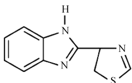
图 5 噻菌灵基本化学结构
