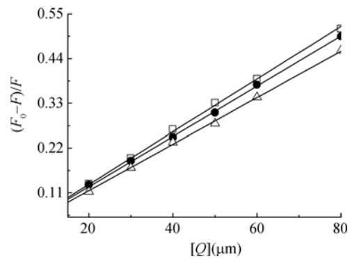
图 3 胶毒素与 BSA 结合的 Stern-Volmer 线性图
