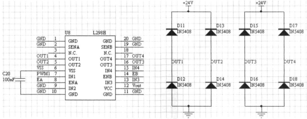
图 3 L298 电机驱动电路
