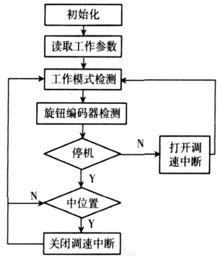
图 6 主程序流程图 Fig.6 Flow chart of main program
