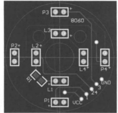
图 4 摆动位置检测集成电路板
