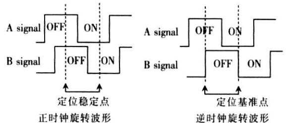
图 5 旋钮编码器输出波形
