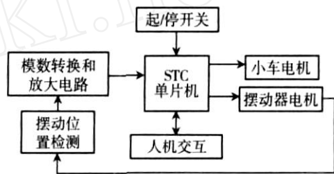
图 2 系统原理框图
