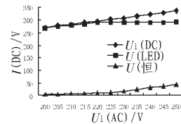
图5 输入电压 U_i (AC)变化对电路的影响
