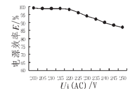
图6 输入电压 U_i (AC)变化与电源效率的关系
