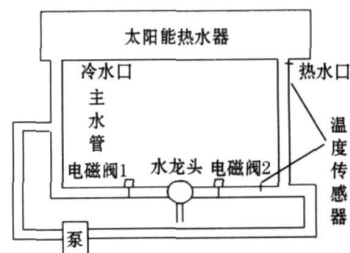
图 1 装置整体结构原理
