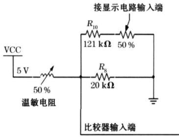
图 4 转换电路
