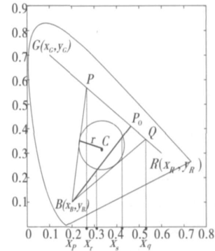
图 2 配色算法示意图
