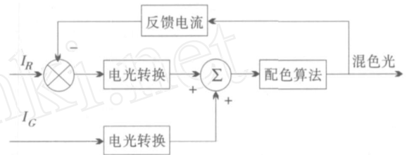
图1 RG-LEDs 配色模型
