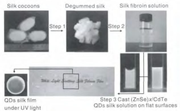
图4 量子点功能化的白光蚕丝薄膜制作过程示意图 [38]
