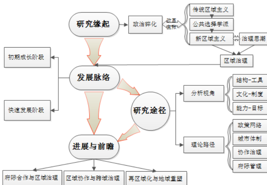
图 1：研究框架图
