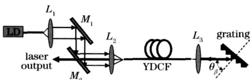
图 1 可调谐掺镱双包层光纤激光器示意图
