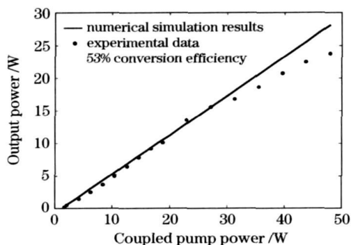
图5 调谐波长为1089 nm时的输出功率特性曲线
