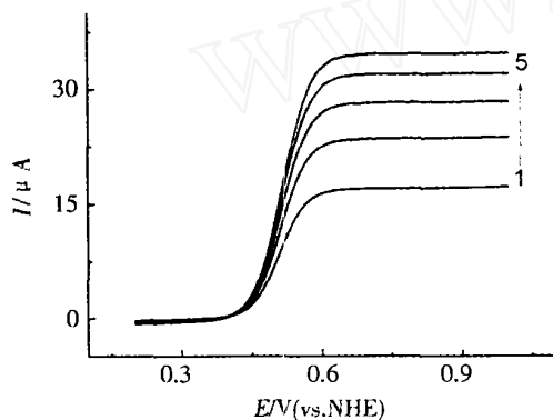
图 1 二茂铁在旋转玻碳电极上的伏安曲线 Fig 1 Voltammetric curves of the ferrocene on GC electrode with different rotation rate rotation rate N/(r \cdot \text{min}^{-1}) : 1) 300, 2) 600, 3) 900, 4) 1200, 5) 1500
