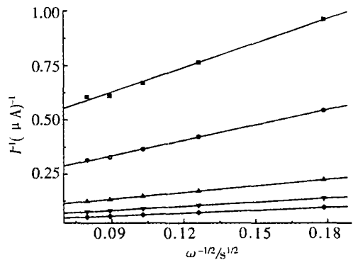
图 2 由图 1 获得的 I^{-1} \sim \omega^{-1/2} 变化关系 Fig 2 Plots of I^{-1} against with the data from Fig 1 E/V : 0.43, 0.45, 0.48, 0.50, 0.52
