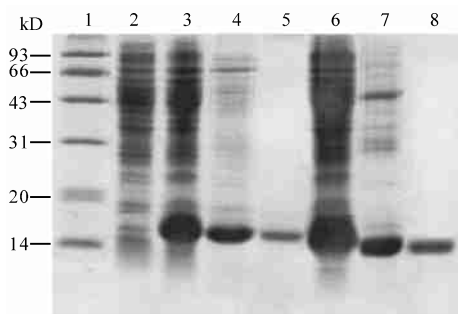
图 2 MA18/7 抗体可变区片段的 SDS-PAGE
