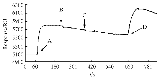
图 3 MA18/7 小分子抗体与 pre-S1 抗原的结合曲线
