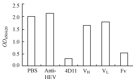
图 4 MA18/7 小分子抗体对单抗 4D11 与抗原结合的竞争
