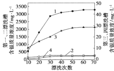
数字标号即漂洗槽编号
