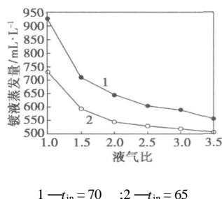
图 5 液气比对镀液蒸发速率的影响
