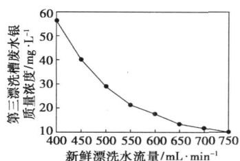
图 4 新鲜漂洗水流量对第三漂洗槽含银量的影响
