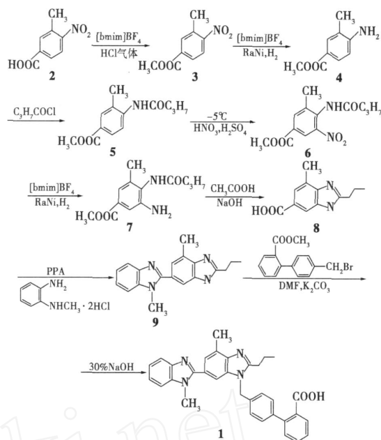
图 3 替米沙坦的合成路线
