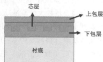
图 3 掩埋条形波导结构示意图
