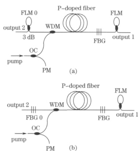
图 1 掺磷 RFL 实验装置示意图
