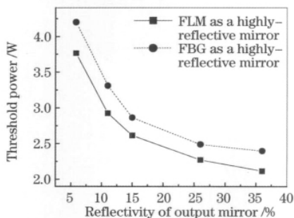
图 4 使用不同反射率输出镜情况下的激光振荡阈值 Fig. 4 Laser threshold with different reflectivities of output mirrors
