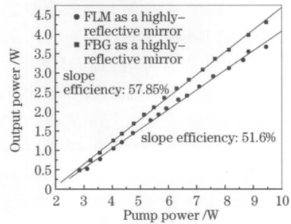
图 5 输出镜反射率为 15% 时激光输出功率与抽运功率的关系
