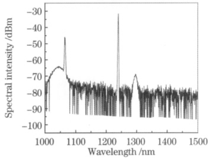
图 2 抽运功率为 6 W 时的典型输出光谱
