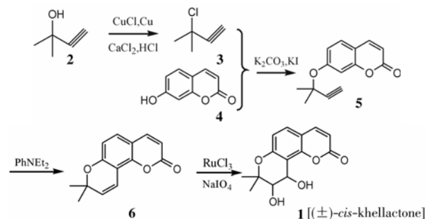
图 1 顺式凯林内酯的合成路线
